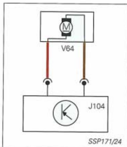
J 104 Steuergerät für ABS/EDS
